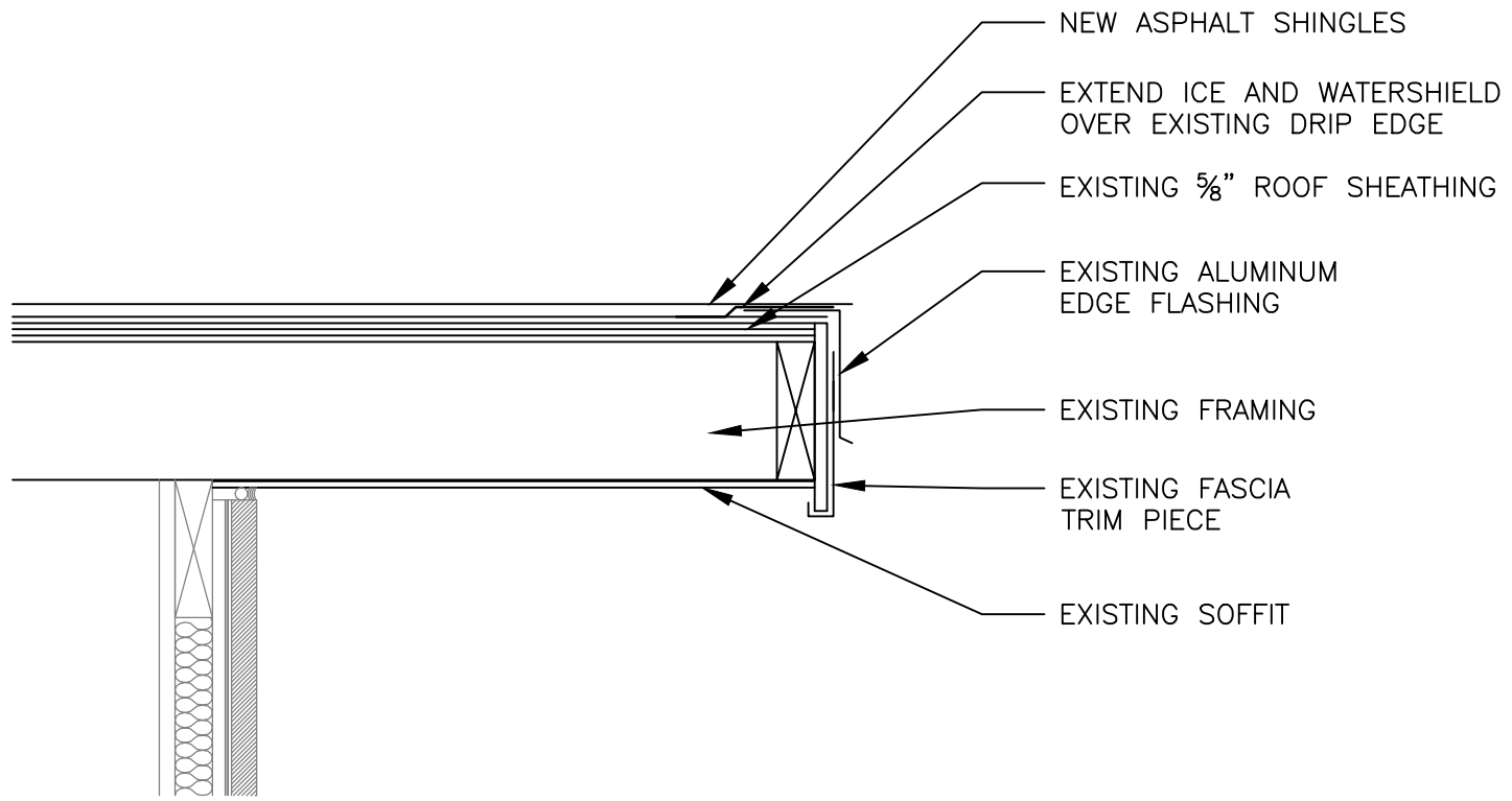
9 RAKE DETAIL A-500 NTS
